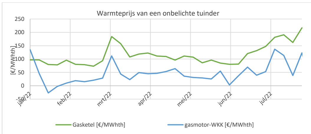
Figuur 2 Warmteprijs van een onbelichte tuinder, op basis van commodity prijzen
