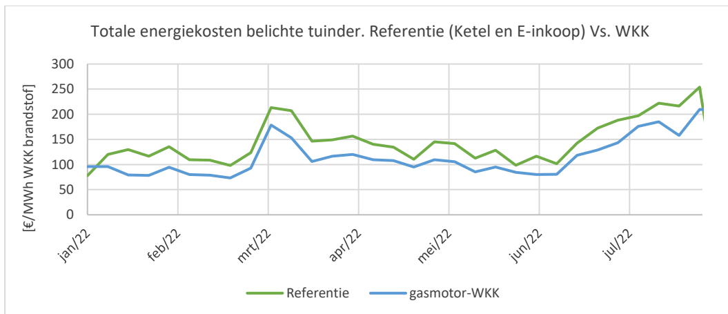
Figuur 3- Totale energiekosten belichte tuinder. Referentie (Ketel en E-inkoop) versus WKK, op basis van commodity prijzen
