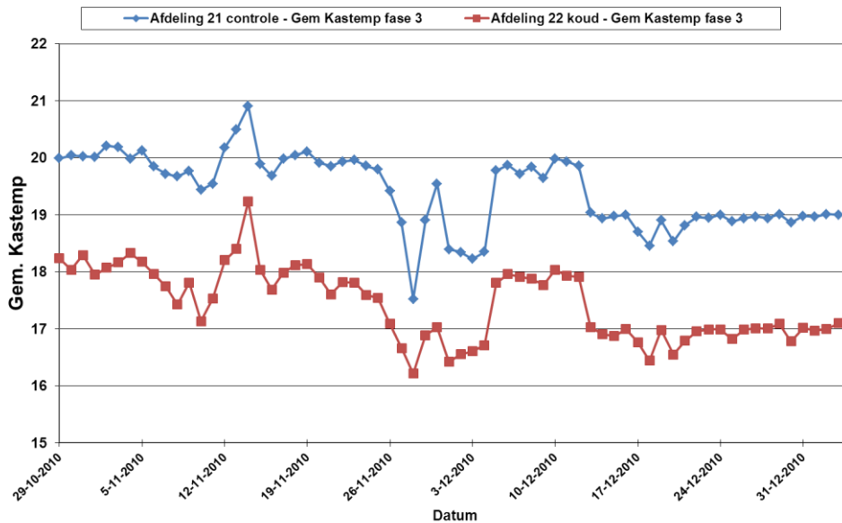
Figuur 8 Gemiddelde kasttemperatuur fase 3; Scherm dicht, belichting uit
