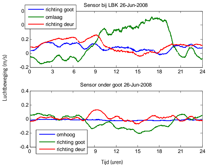
Figuur 17. Luchtbewegingen vóór aanpassing van de uitblaasmonden, gemeten op 26 juni 2008. Luchtbeweging was hevig en voornamelijk neerwaarts gericht nabij de JSK, zoals te zien in de bovenste grafiek (Sensor bij LBK). Luchtbeweging onder de goten, zoals te zien in de onderste grafiek (Sensor onder goot) was veel minder dan naast de JSK.
