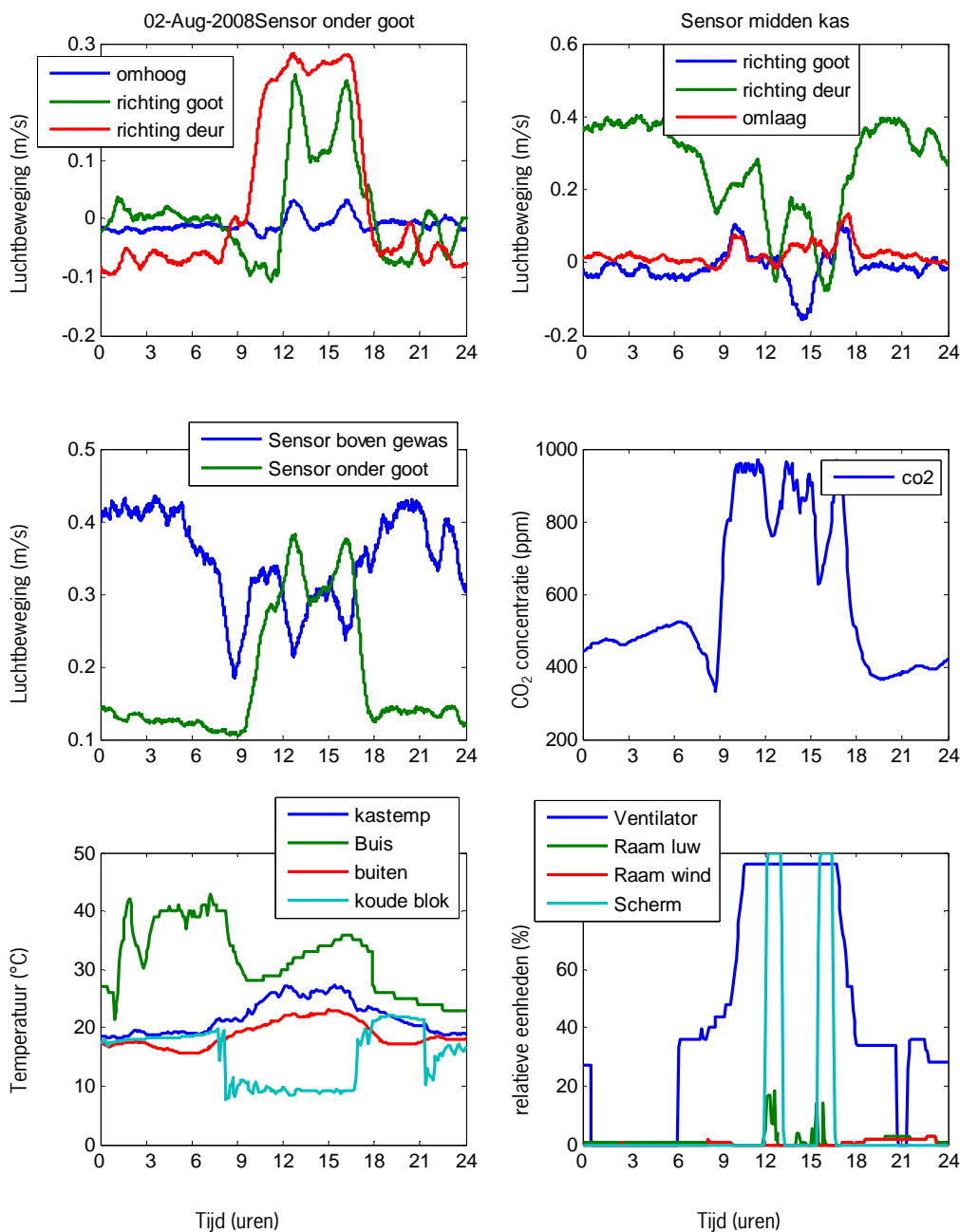
Figuur 19. Lucht bewegingen na de aanpassingen aan de uitblaasmonden, gemeten op 2-08-2008 onder de middelste goot (Sensor onder goot) en boven de kop van het gewas op de middelste goot (Sensor midden kas), wanneer deze bewegingen bekeken worden aan de hand van de veranderingen in de snelheid van de JSK (Ventilator) en de stand van het doek (Scherm), dan is te zien dat zowel boven het gewas als onder de goot veranderingen optreden, zoals eerder waargenomen voor de aanpassingen. Echter, de sensor boven het gewas (Sensor midden kas) laat een duidelijk ander beeld zien dan voor de aanpassingen aan de uitblaasmonden dat aangeeft dat de luchtbewegingen zijn veranderd als gevolg van hiervan.
