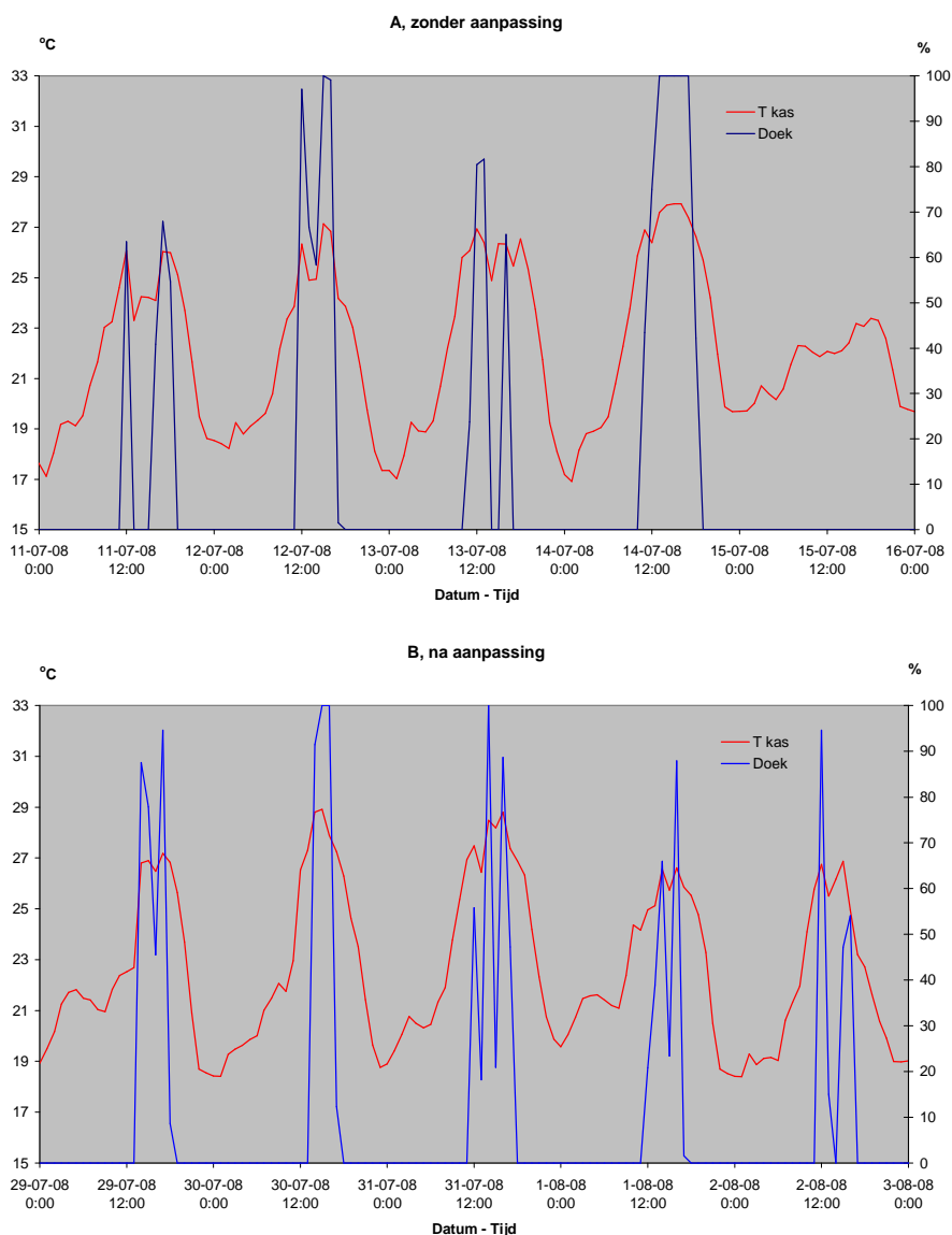
Figuur 8. Overzicht kasttemperatuur ( T , °C, linker as) en doekstand (Doek, %, rechter as) per uur voor de perioden 11-07 tot en met 14-07-2008 (A, zonder aanpassingen aan uitblaasmonden) en 29-07 tot en met 03-08-2008 (B, met aanpassingen)
