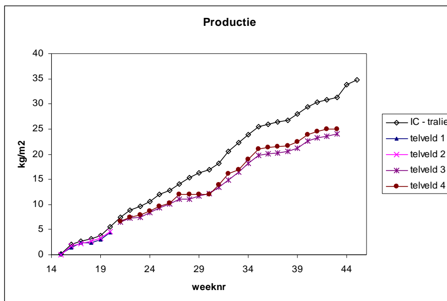
Figuur 21. Cumulatieve productie van de hele tralie (IC - tralie) en van de verschillende telvelden. Tot en met week 20 zijn twee telvelden gebruikt (telveld 1 en telveld 2), waarna twee nieuwe telvelden zijn gebruikt (telveld 3 en telveld 4).
