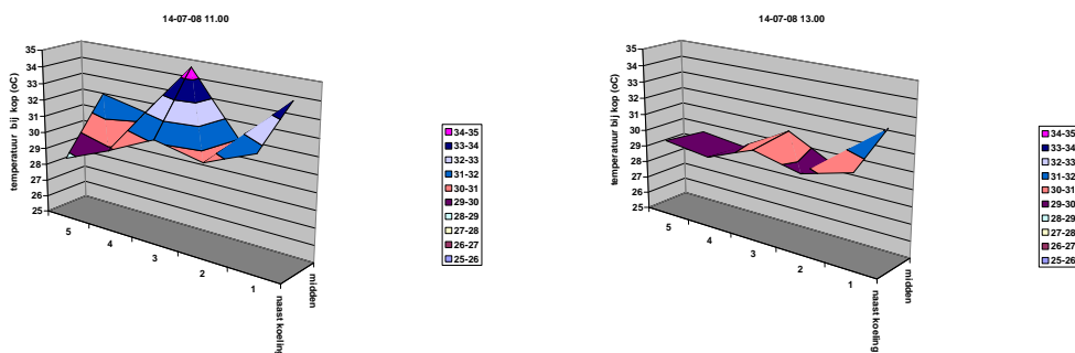
Figuur 10. Verdeling van temperatuur bij de kop op 14-7-2008, vóór aanpassingen van de uitblaasmonden. Er is te zien dat de temperatuur in het gewas op de middelste goot (midden), een hogere waarde heeft in vergelijking met de temperatuur in de kop naast de JSK (naast koeling). (klimaat om 11.00: kas temperatuur 26,8 °C, straling 755 W m -2 , doek stand 43%; klimaat om 13.00: kas temperatuur 27,6 °C, straling 793 W m -2 , doek stand 100%)
