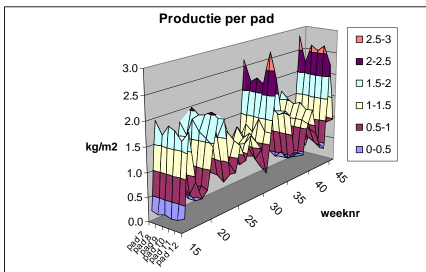
Figuur 20. Productie per week van de paden in de tralie tussen de JSK installatie.
