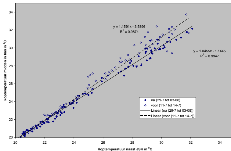
Figuur 9. Relatie tussen de temperatuur bij de kop van de plant naast de JSK en die in de kop van de middelste goot. De temperaturen in de eerste periode, waarbij nog geen aanpassingen gedaan zijn aan de uitblaasmonden laten zien dat er een hogere temperatuur bij de kop in de middelste goot is ( \diamond voor (11-7 tot 14-7)). De relatie tussen de twee temperaturen is iets hoger dan 1 (1.159). Na de aanpassingen van de uitblaasmonden, is te zien dat de temperaturen in het midden minder verschillen van die naast de JSK ( \blacklozen , na (29-7 tot 03-08)). De relatie tussen de twee temperaturen is tevens verbeterd (1.046).
