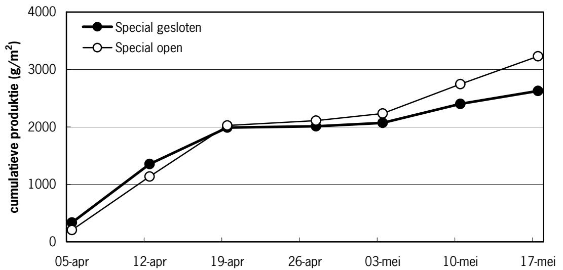
Figuur 2 - Cumulatieve productie (g/m 2 ) bij een gesloten en geopend scherm bij het paprikaras Special van de vroege productie.
