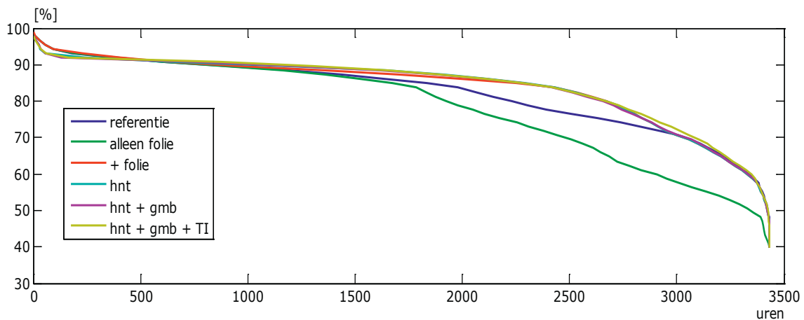
Figuur 15. Jaarbelastingduurkromme van de berekende RV's voor de referentie en 5 scenario's in de periode 19 januari tot en met 6 juni.
