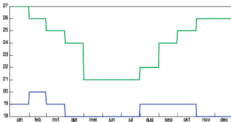
Figuur 7.: Weergave van de ventilatielijn (groen) en de stooklijn (blauw) in referentieteelt.
