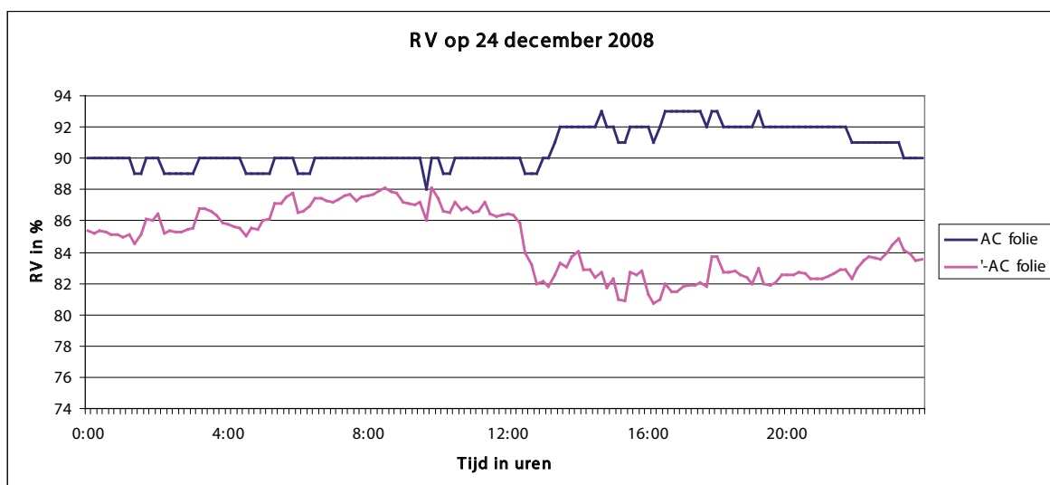
Figuur 15.: RV verloop op een willekeurige decemberdag in twee praktijkbedrijven in 2008-2009, waarvan een bedrijf met foliescherf (AC folie) en de andere zonder foliescherf ('- AC folie). Uit Warmenhoven en García, 2009.
