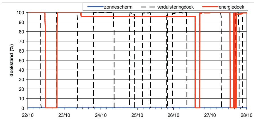
Figuur 6. BuiSTEMPERatuur, ventilator en doekstanden in de meetperiode.
