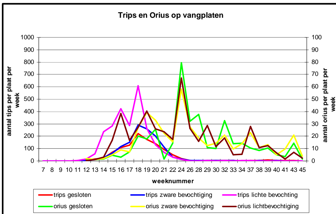
Figuur 1 Trips en de bestrijder Orius gescout op vangplaten
