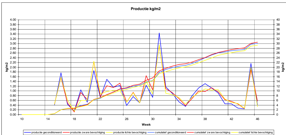
Figuur 4-1 Verloop van de productie in kg/m 2 per week en cumulatief
