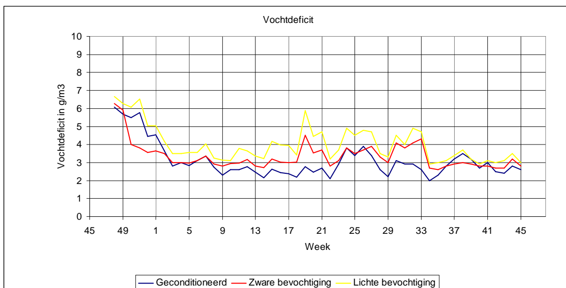
Figuur 5-2 Het gemiddelde vochtdeficit per week
