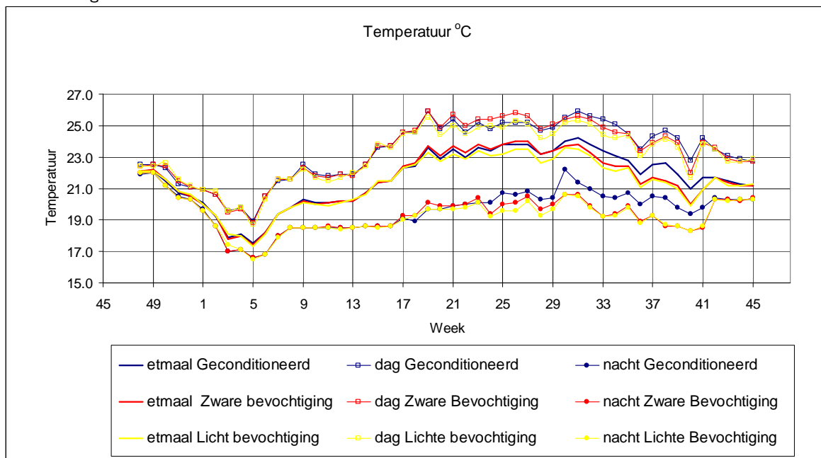
Figuur 5-1 Verloop van de gemiddelde temperatuur per afdeling. De temperaturen worden gegeven per etmaal, voor de uren overdag en de uren in de nacht. De dag temperaturen zijn de drie bovenste lijnen en de nacht temperaturen de drie onderste lijnen.
