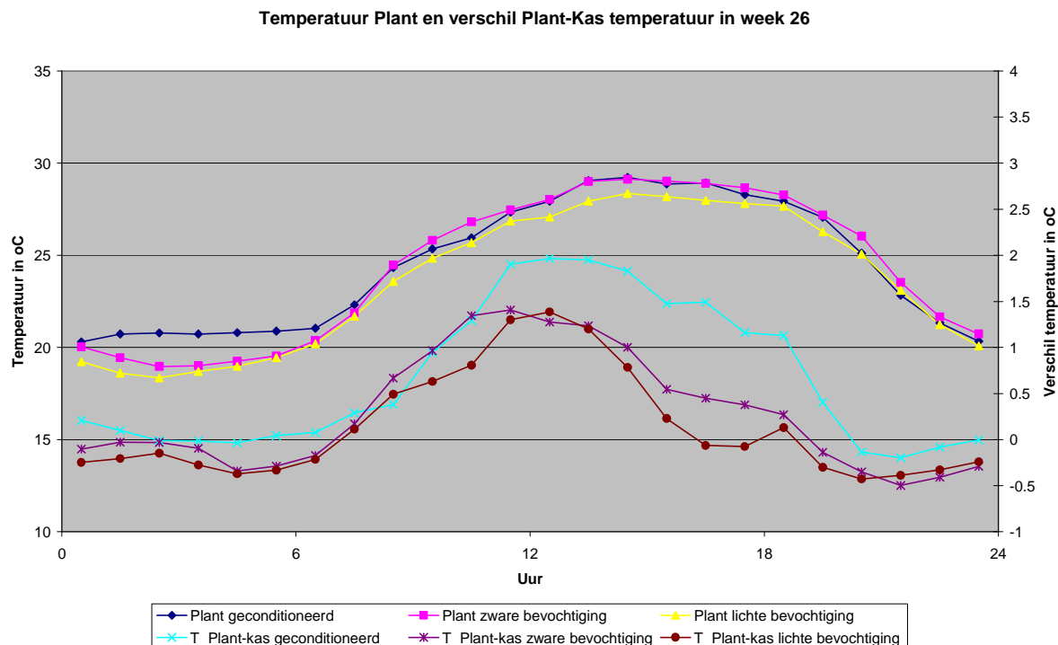
Figuur 6 Planttemperatuur en verschil Plant-Kas temperatuur in week 26.
