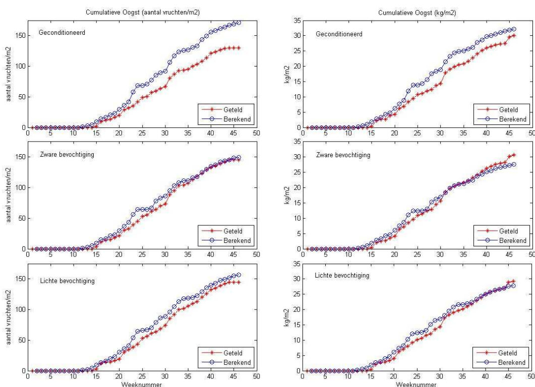
Figuur 4-3 Cumulatieve oogst per week per netto teeltoppervlak voor drie behandelingen. De getelde oogst in telvelden (Geteld, rode lijn en symbolen) en door Papigrow berekende oogst aan de hand van het gerealiseerde klimaat (Berekend, blauwe lijn en symbolen) zijn per kas weergegeven. Hierbij is er onderscheid gemaakt tussen de oogst geteld in het aantal vruchten en het gewicht ( \text{kg} ) per \text{m}^2 .
