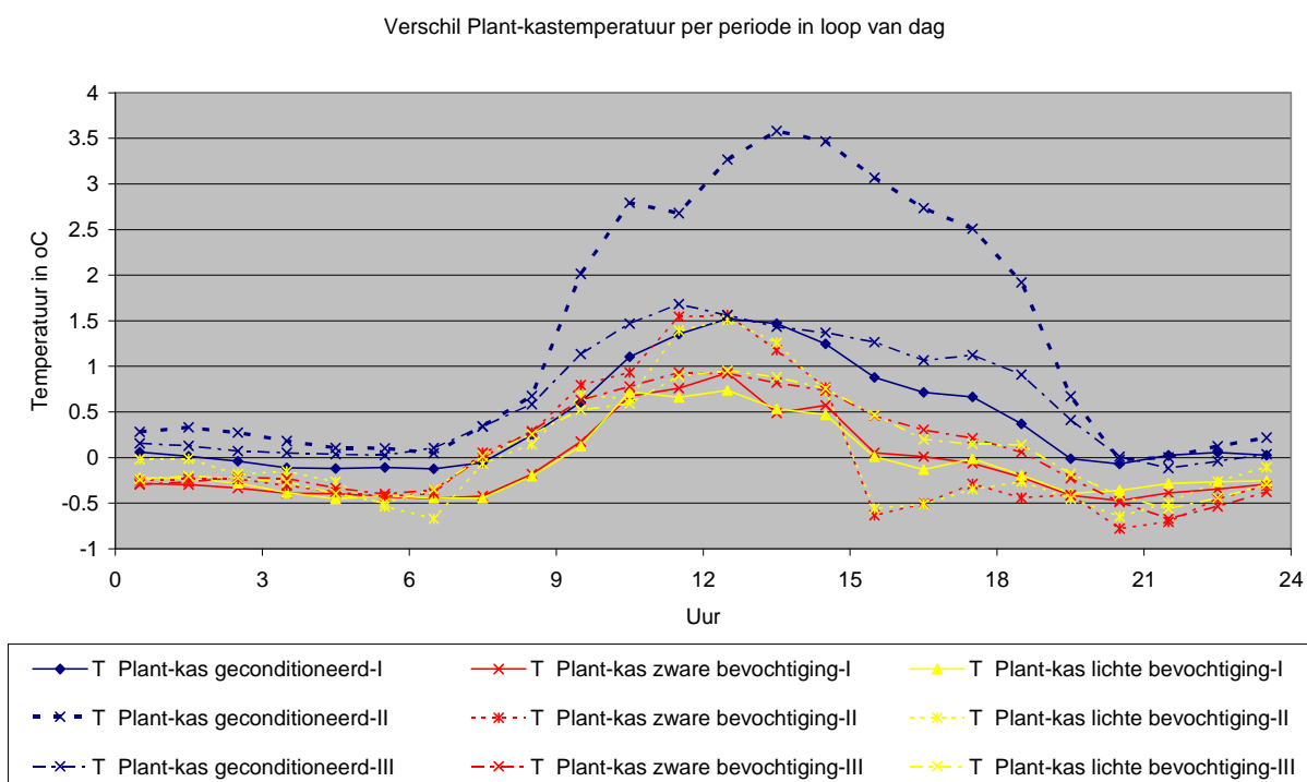
Figuur 5 Planttemperatuur en verschil Plant-Kastemperatuur in drie perioden rond begin mei.
