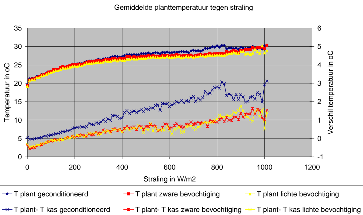
Figuur 3 Plant temperatuur tegen straling in de periode april-juni
