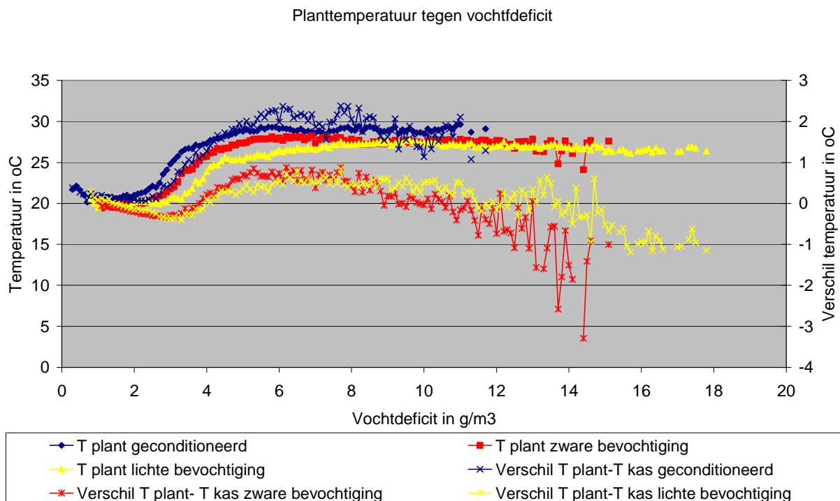
Figuur 4 Planttemperatuur tegen vochtdeficit in de periode april - juni
