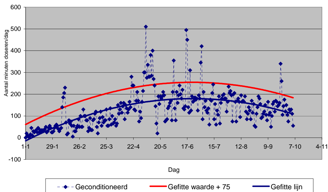
Figuur 2 CO 2 dosering in de geconditioneerde kas.
