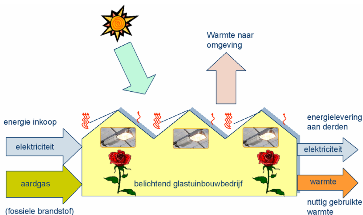
Figuur S.1 Schematische voorstelling van een belichtend glastuinbouwbedrijf met de belangrijkste intredende en uitredende energiestromen
