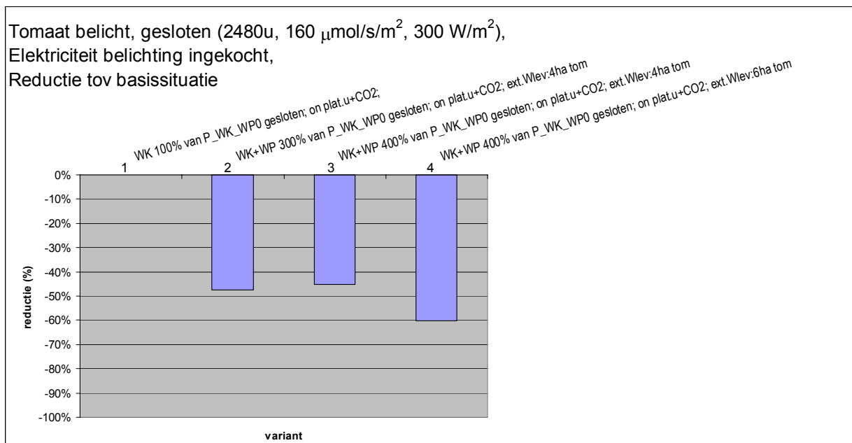
Figuur 3.7 Procentuele besparing op energieverbruik bij verschillende hoeveelheden externe warmtelevering in het geval van semi-gesloten, belichte tomaat (centrale-rendement: 45% o.w.)
