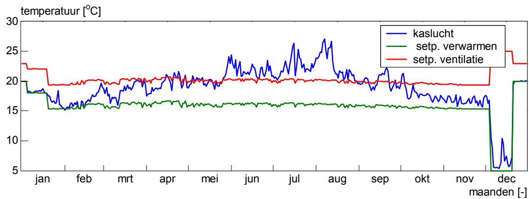
Figuur 8 Daggemiddelde gerealiseerde kasluchttemperatuur, setpoint verwarmen en setpoint ventilatie.
