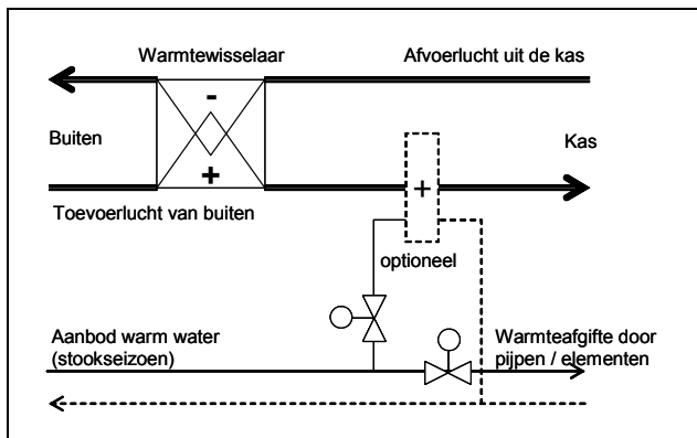
Figuur 1 Zelfstandige gebalanceerde ventilatie met warmteterugwinning.
