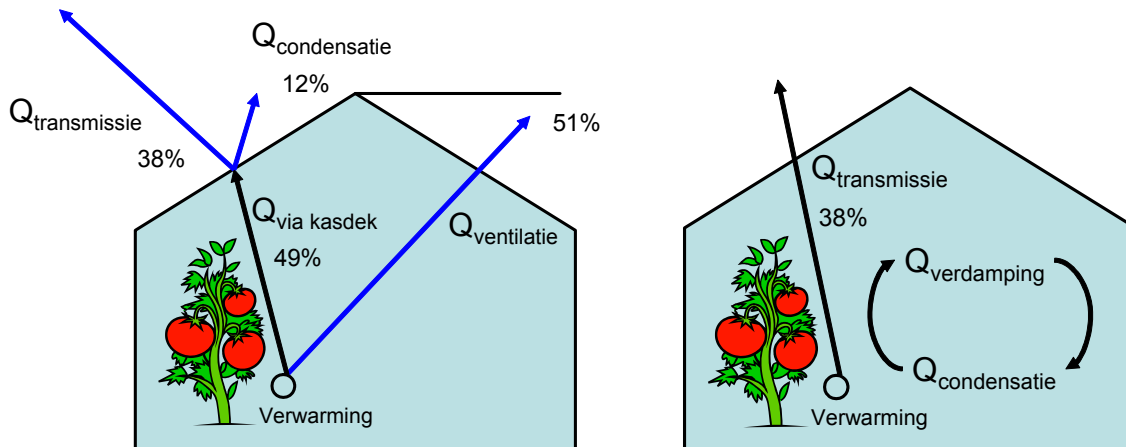
Jaargemiddelde warmteafvoer door condensatie en ventilatie, voor zover die warmte door de verwarming wordt ingebracht, tomat, enkel glas, simulatie KasPro.
