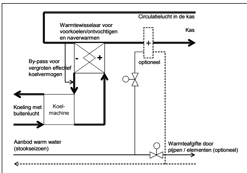
Figuur 6 Uitkoelen van vocht met koelmachine.
