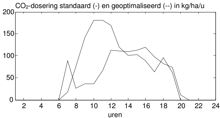
Figuur 4.3 Verloop van de CO 2 -dosering in de standaardkas (getrokken lijn) en in de kas met de optimaliserende regelaar (gestreept) dat nodig is om in beide situaties tot dezelfde fotosynthese te komen.
