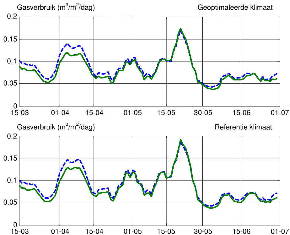
Figuur 7.6 Dagelijks gasverbruik indien het gemeten klimaat in een grote kas zou zijn gerealiseerd (getrokken lijn) en zoals dat in de onderzoekkas is opgetreden (onderbroken lijn). In de bovenste grafiek staat deze vergelijking afgebeeld voor het geoptimaliseerde klimaat en in de onderste grafiek is dit gedaan voor het referentieklimaat.
