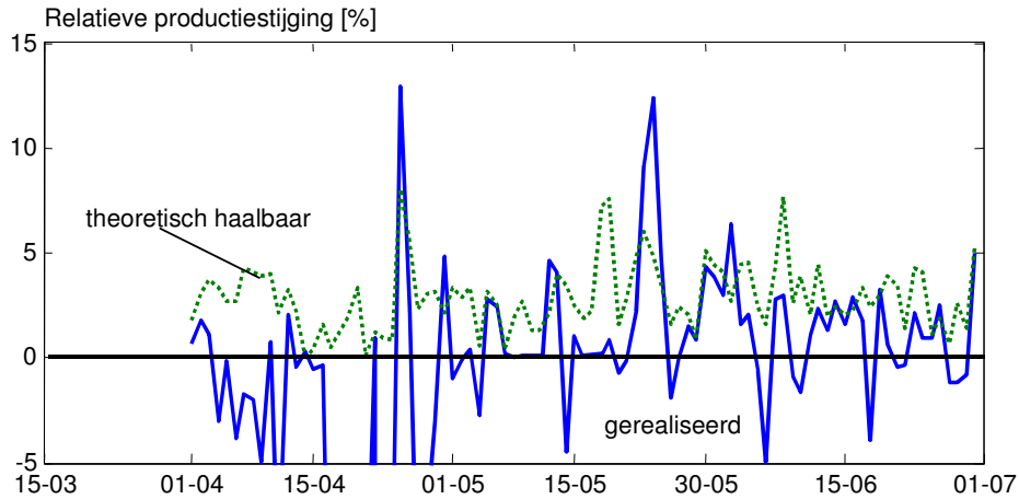
Figuur 7.8 Relatieve berekende productietoename in de afdeling waarin de optimaliserende regeling werd gebruikt ten opzichte van de referentie-afdeling (getrokken lijn) en de achteraf berekende theoretisch haalbare relatieve productiestijging (gestippelde lijn). De regeling werd half april geïmplementeerd en functioneerde vanaf mei in softwarematige zin naar behoren.
