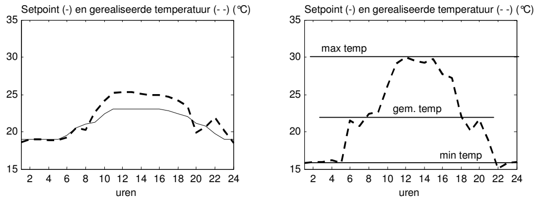
Figuur 4.1 Typisch verloop van het kasklimaatsetpoint (getrokken lijn) en de gerealiseerde temperatuur (gestreepte lijn) in de referentie teelt (links) en volgens het energie-zuinige algoritme (rechts) op een dag in het voorjaar (10 april in het SEL-jaar).
