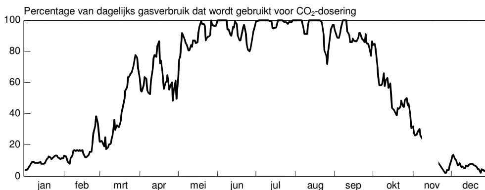
Figuur 3.4 Percentage van het dagelijks gasverbruik dat wordt ingezet voor CO 2 -dosering.
