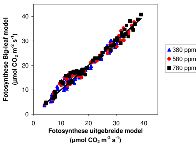
Figuur 2.1 Bruto fotosynthesesnelheid berekend door het Big-leaf model uitgezet tegen de bruto fotosynthesesnelheid berekend door het uitgebreide model bij 3 CO 2 concentraties (zie legenda).
