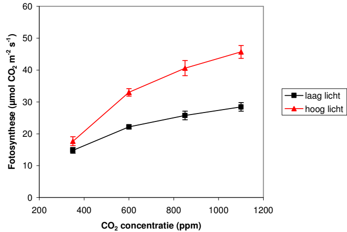
Figuur 9.2 Netto fotosynthesesnelheid van paprikabladeren bij een reeks CO 2 concentraties in de bladkamer gemeten bij hoog (1500 µmol m -2 s -1 ) en laag licht (250 µmol m -2 s -1 ) en een temperatuur van 25 °C. Meetpunten zijn het gemiddelde van 12 meetwaarden met de sem.
