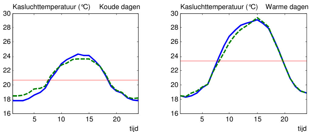
Figuur 7.4 Gemiddeld verloop van de kasluchttemperatuur op 48 relatief koude dagen en 32 relatief warme dagen in de afdeling waar temperatuurintegratie gebruikt wordt (getrokken lijn) en in de referentieafdeling (onderbroken lijn). De horizontale lijn markeert de etmaalgemiddelde temperatuur
