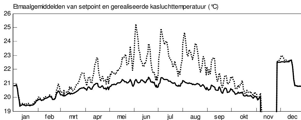
Figuur 3.1 Verloop van de etmaal gemiddelde kasluchttemperatuur (gestreept) en de temperatuur die op de klimaatcomputer is ingesteld (getrokken lijn) over de teeltperiode van een standaard paprikateelt.
