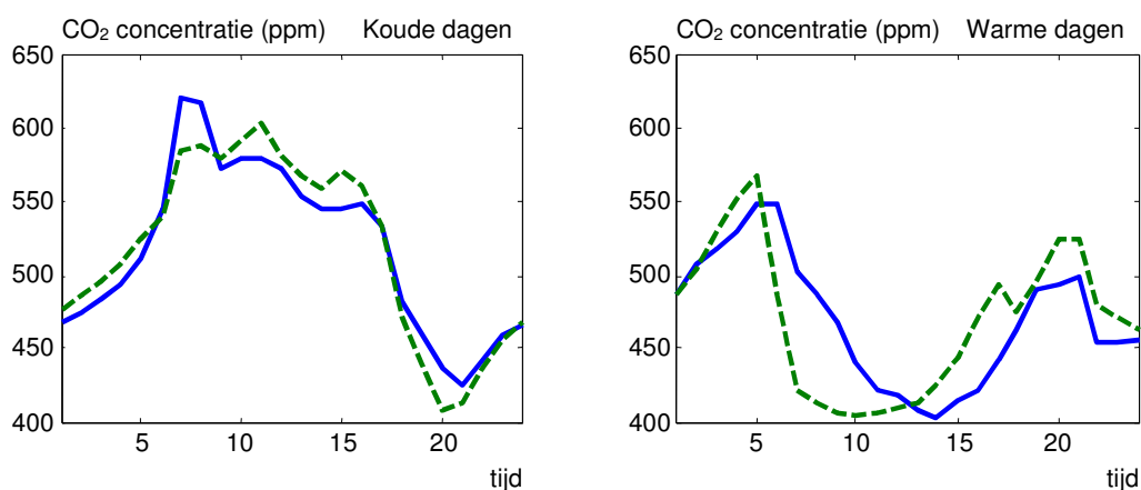
Figuur 7.7 Gemiddeld verloop van de CO 2 -concentratie in de kas op 48 relatief koude dagen en 32 relatief warme dagen in de afdeling waar de dosering werd geoptimaliseerd (getrokken lijn) en in de referentieafdeling (onderbroken lijn).
