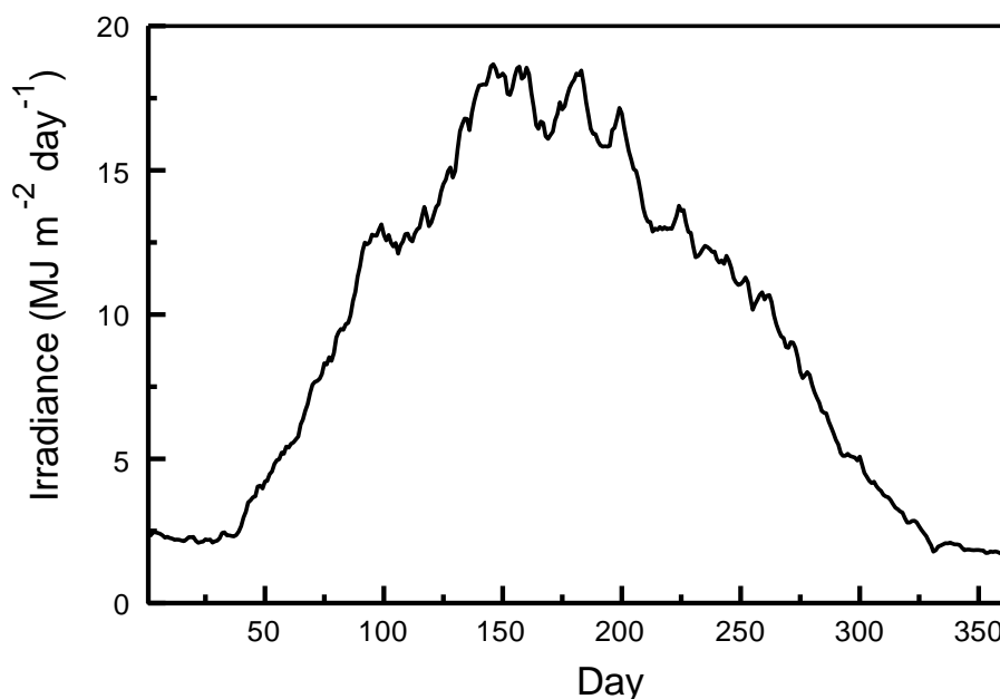
Fig. 3. Stralingssom van het natuurlijk daglicht over het jaar van het zogenaamde SEL-year uit de periode 2000-2007 volgens de methode van Breuer & van de Braak, 1989.
