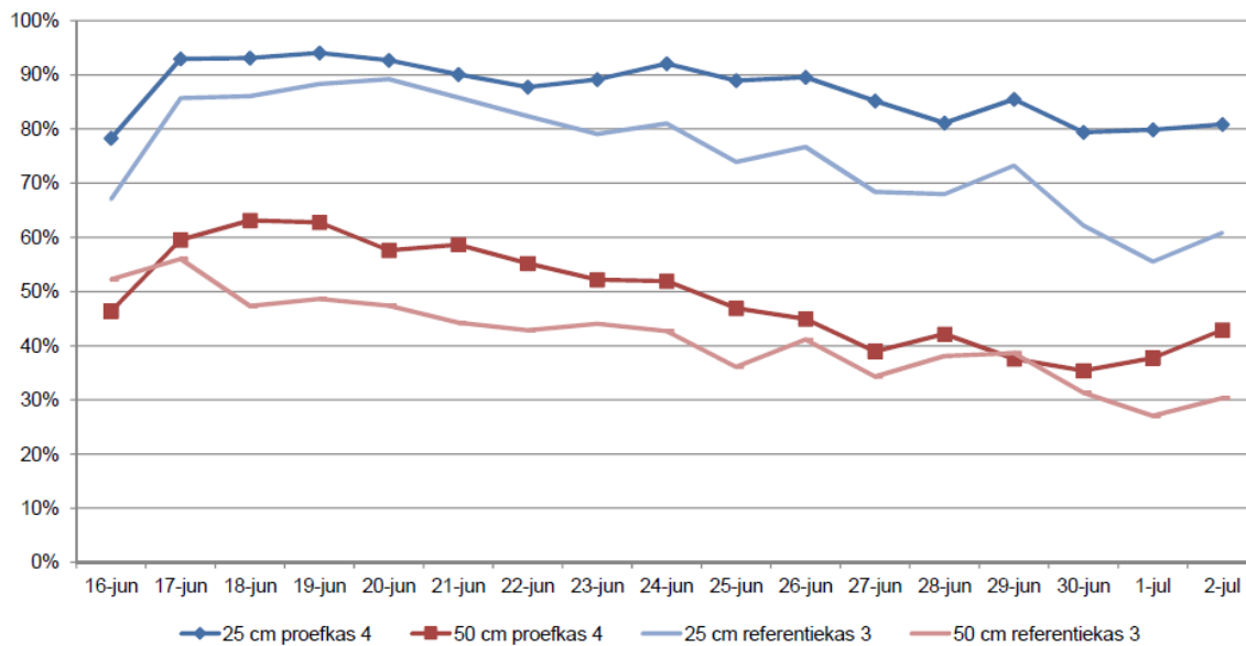
lichtverdeling 16 juni - 3 juli 2015 proefkas 3 en 4 - 25 en 50 cm onder de kop
