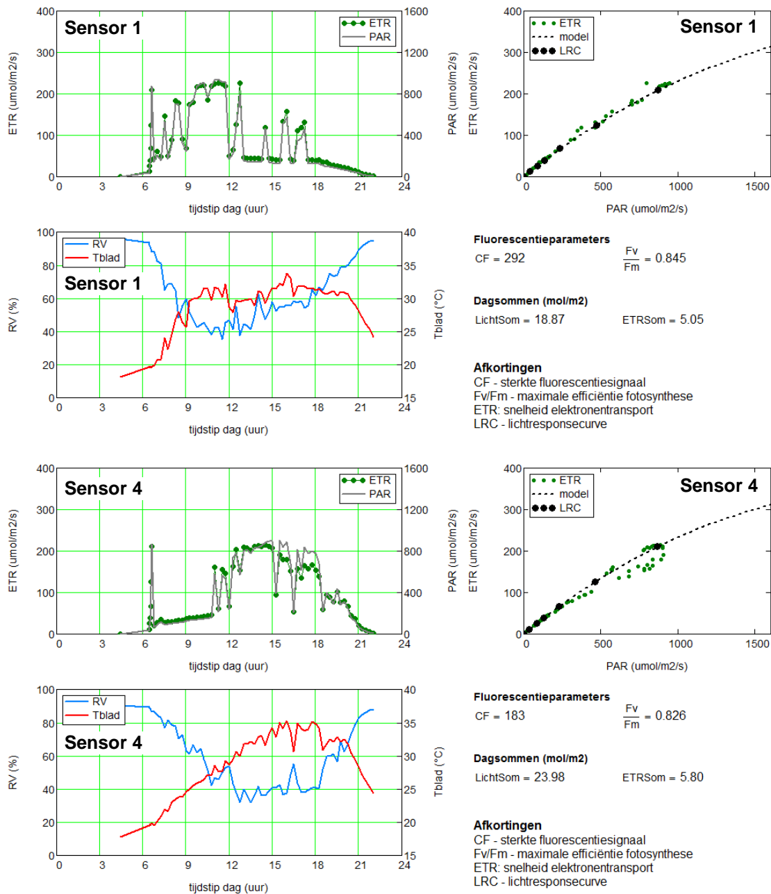
Figuur 4.7.9. Links: verloop van PAR, ETR, bladtemperatuur en RV van sensor 1 (boven) en sensor 4 (onder) op 30 juni in kas 4 (HNT). Rechts: lichtresponscurve en ETR uitgezet als functie van de PAR.
