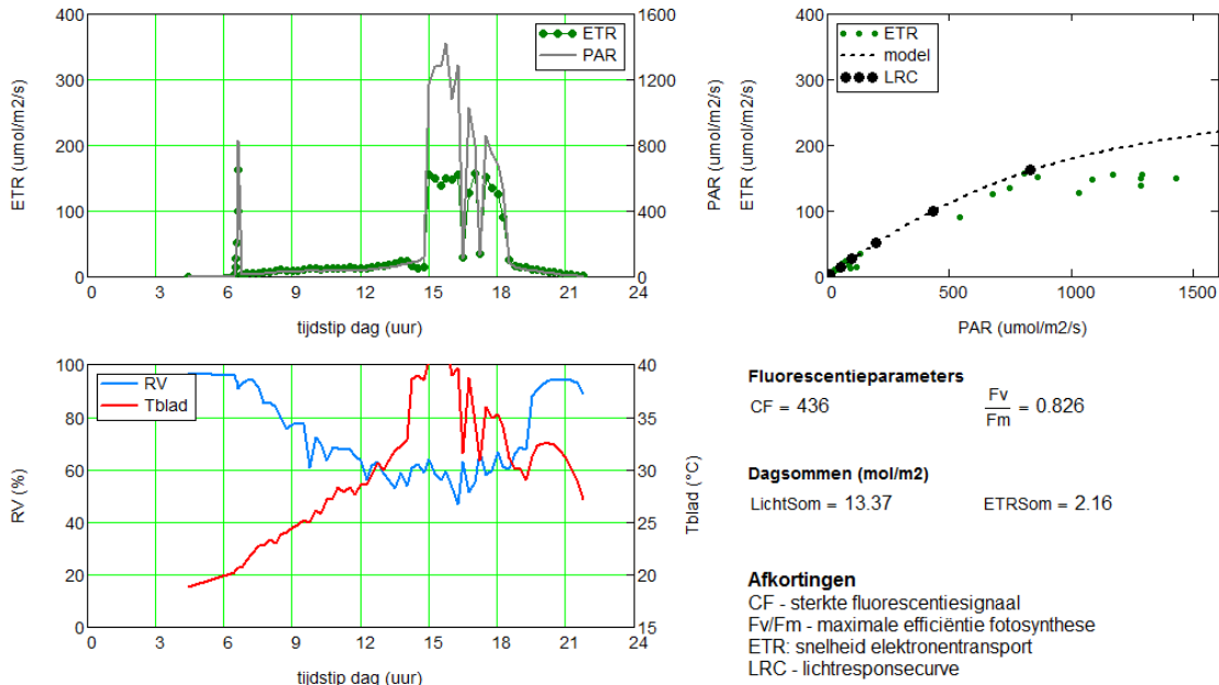
Figuur 4.7.7. Verloop van PAR en ETR (linksboven) en bladtemperatuur en RV (linksonder) van sensor 2 (midden in gewas) op 1 juli in kas 3 (Referentie). Rechtsboven de metingen van de lichtresponsecurve en de ETR uitgezet als functie van de PAR.
