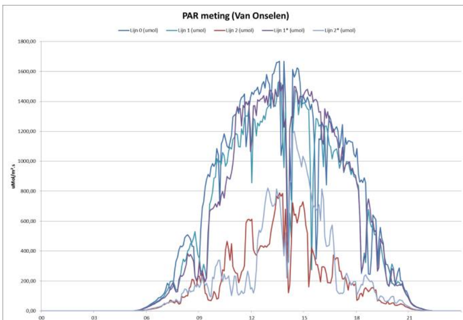
10-7-2015: Lichtdoordringing zonnige dag
