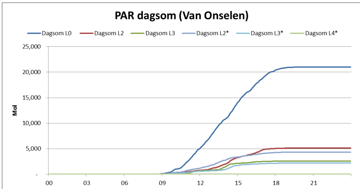
Grafiek: Dagsommen 20-9-2015 onder in het gewas bij Van Onselen
