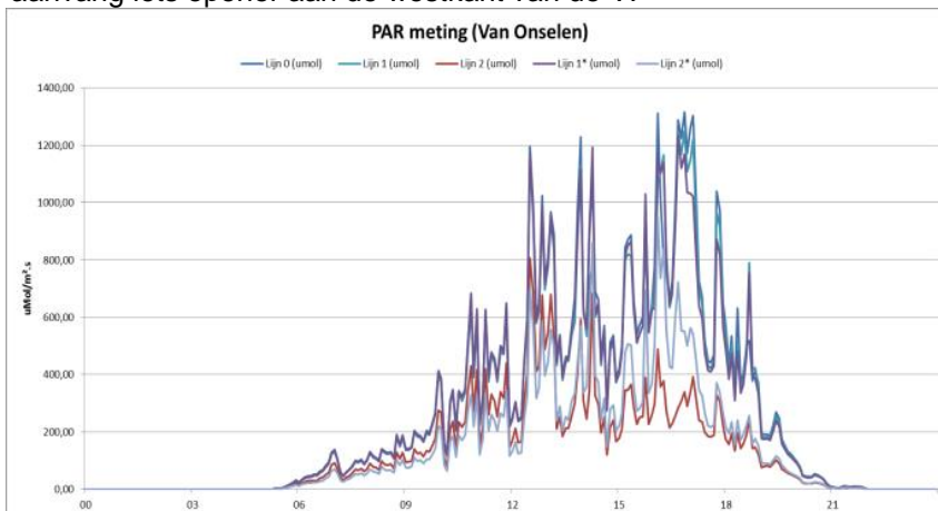
8-7-2015: Lichtdoordringing bewolkte dag
