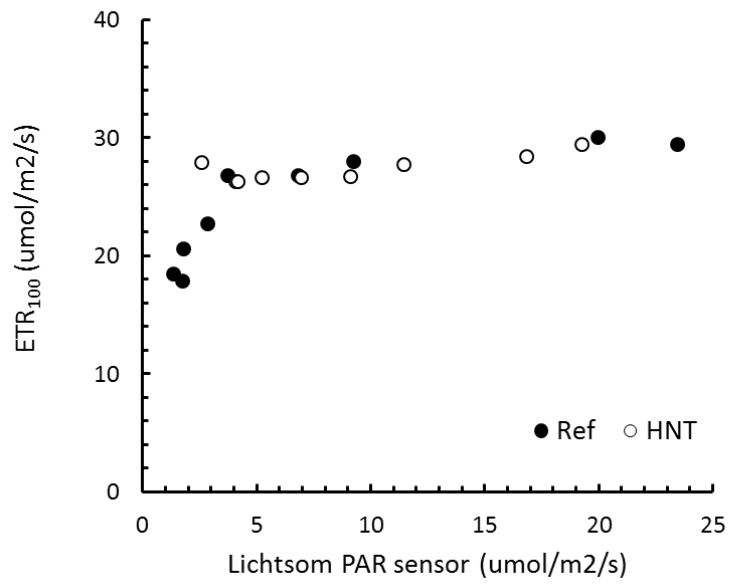
Figuur 4.7.12. De ETR bij 100 \mu\text{mol}\cdot\text{m}^{-2}\cdot\text{s}^{-1} van de drie bladlagen op 23, 26 en 30 juni 2015. De ETR 100 is berekend als het gemiddelde van de potentiële ETR van de twee sensoren per gewaslaag.
