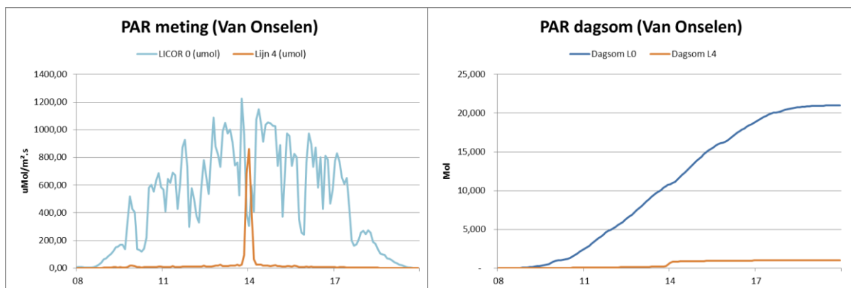
Grafiek: Lichtmeting in het pad (25-9-2015)
