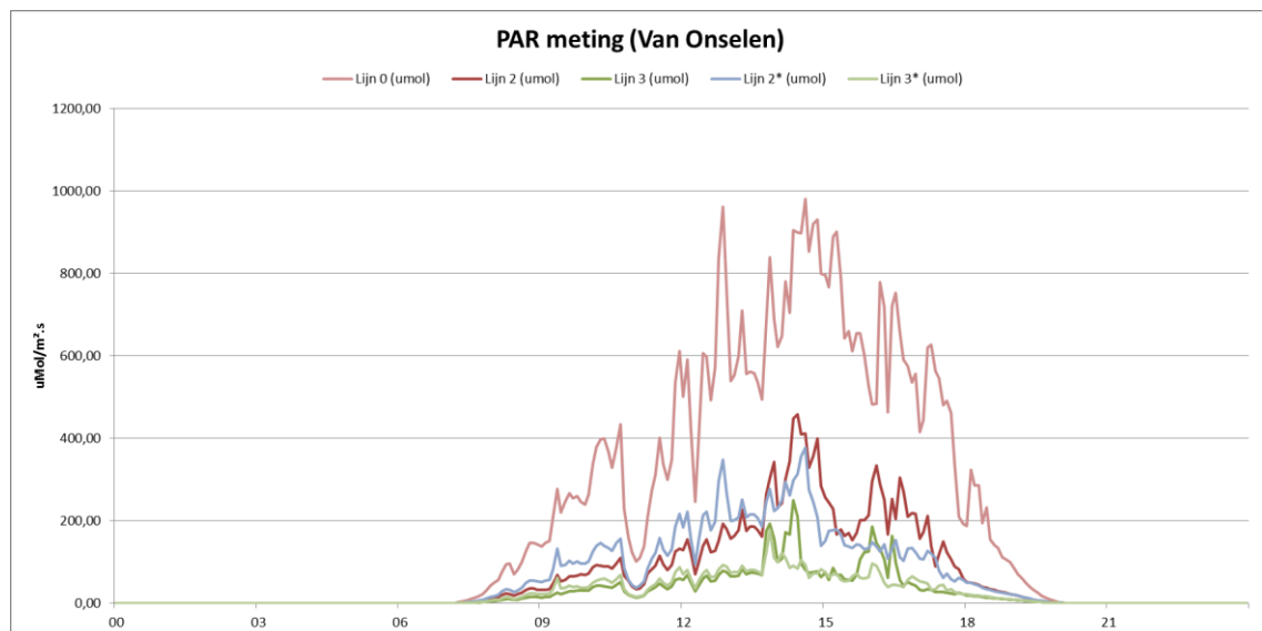
Grafiek: Lichtdoordringing 20-9-2015 onder in het gewas bij Van Onselen
