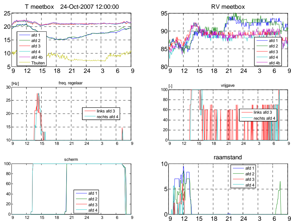
Figuur 20 Klimaat en instellingen van het system op 24 oktober 2007. Linksonder staan de temperaturen in de verschillende afdelingen met de buitentemperatuur, daarnaast staat de relatieve luchtvochtigheid in deze afdelingen, daaronder staat de frequentie waarmee de ventilatoren worden aangestuurd met daarnaast een indicatie wanneer het systeem in werking was (bij waardes hoger dan 0), linksonder staat een grafiek waar de schermstand van de verschillende afdelingen te zien is met daarnaast de raamstand in de verschillende afdelingen.
