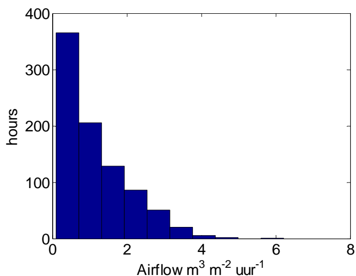
Figuur 8 Aantal uren per jaar dat een specifiek luchtdebiet nodig is in m 3 m -2 uur -1 .
