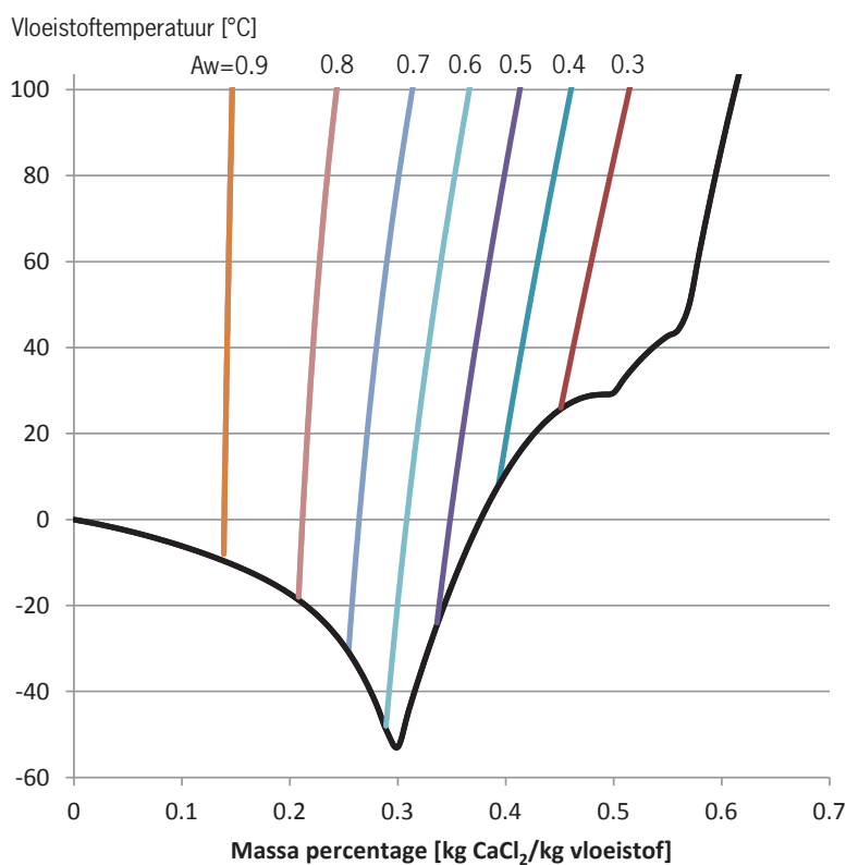
Figuur 6.3. Diagram met de wateractiviteit en oplosbaarheidsgrenzen van een oplossing van CaCl 2 (naar Conde, 2002)
