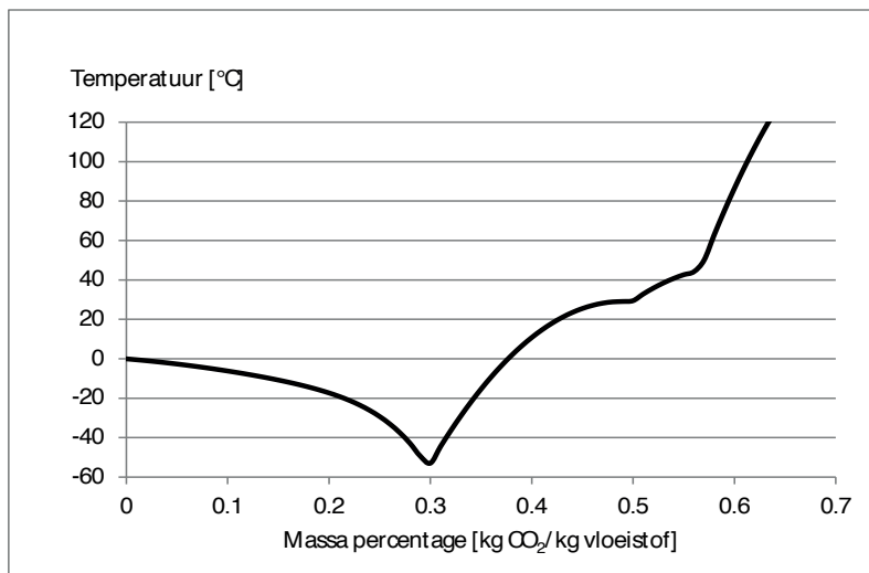
Figuur 6.2. Temperatuur waarboven een oplossing van CaCl 2 vloeibaar is
