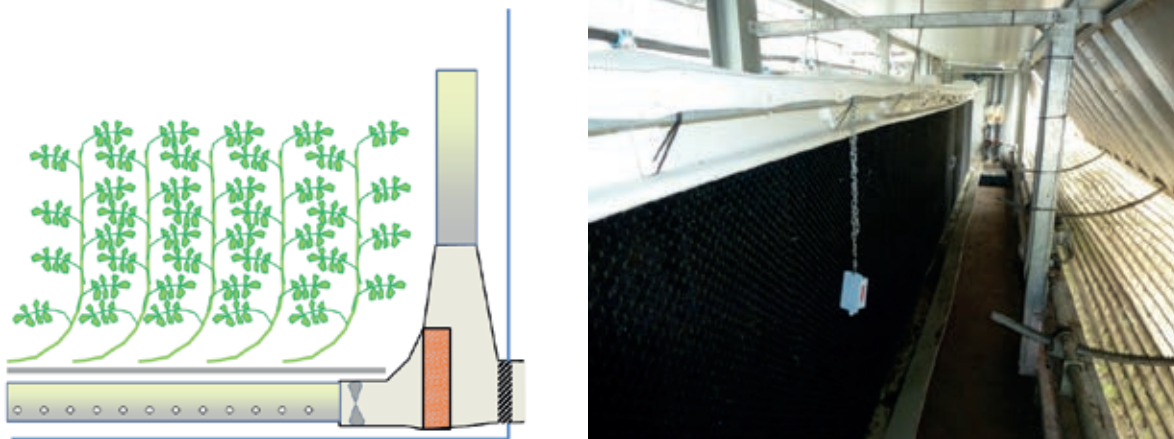
Figuur 6.4. Het vocht- en warmtewisselende oppervlak dat in de schets als rood blok wordt weergegeven is in de praktijk een open structuur waar de hygroscopische vloeistof langs het oppervlak van de structuur stroomt en de lucht door de open ruimten.
