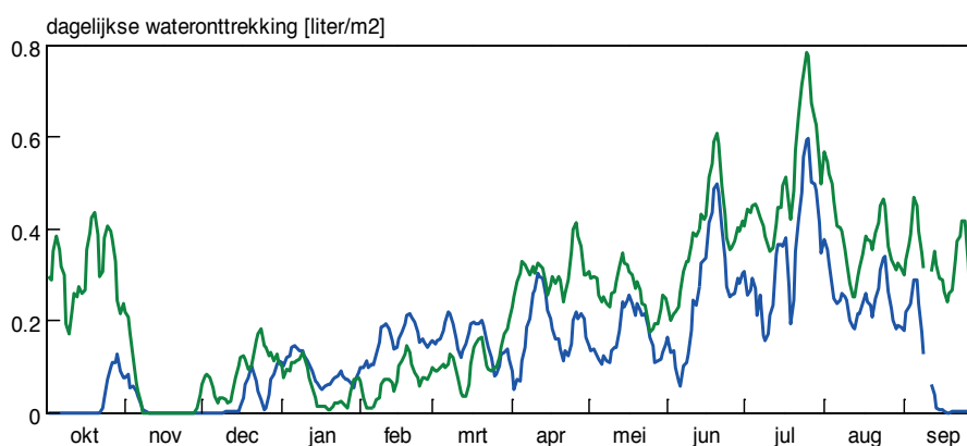
Figuur 4.6. Hoeveelheid ontvochtiging in de Next Generation Semigesloten Kas tijdens bedrijf van de luchtbehandelingskast in het afgelopen jaar (blauwe lijn) en indien de installatie het hele jaar zou hebben gewerkt zoals bedoeld. (Voor een betere leesbaarheid zijn de lijnen afgevlakt met een 5-daags voortschrijdend gemiddelde filter)
