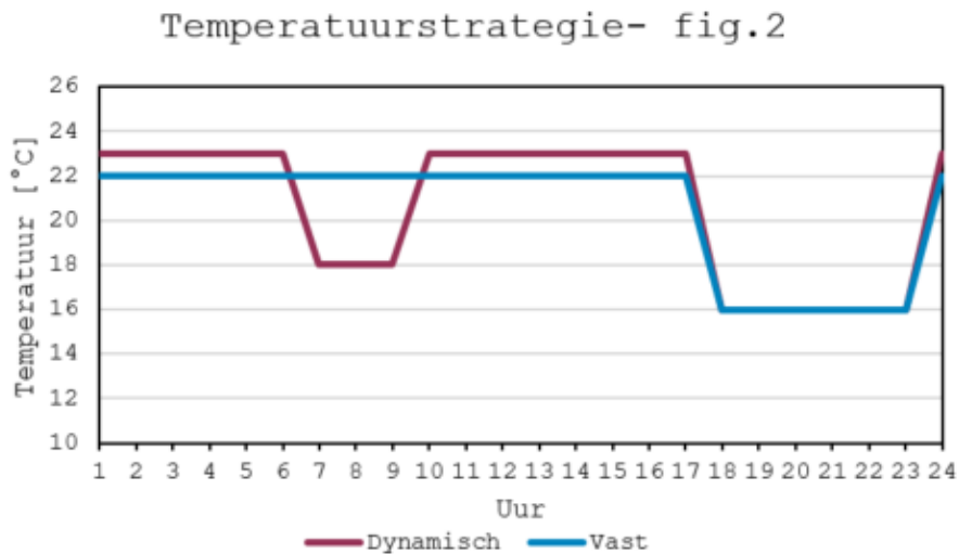
Figuur 2. Grafische weergave van de verwarmingstemperatuurstrategie. De gewenste temperatuur is gekoppeld aan de lichtintensiteit, waarbij de dynamische kas in de dimperiode (6:00-9:00) mag afkoelen om buisinput zo veel mogelijk te voorkomen.
