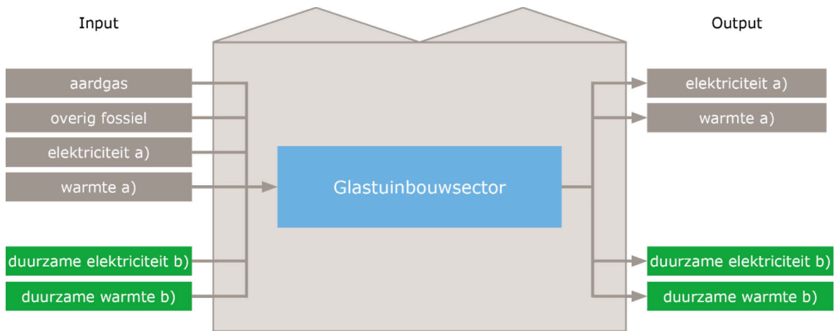
Figuur 2.4 Energie-input en -output glastuinbouw
